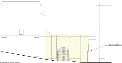
EXISTING ELEVATION Scale: 1:100
