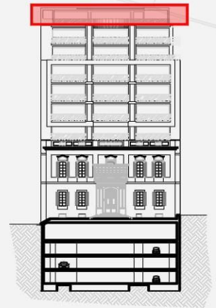
Elevation
