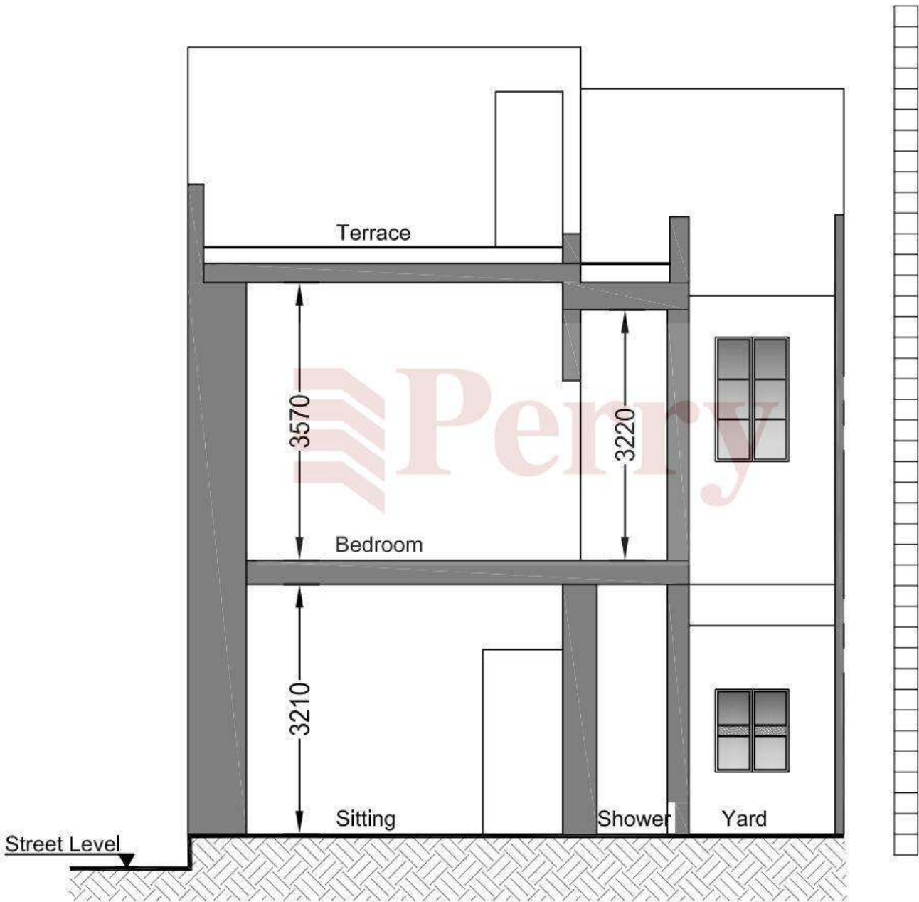
SECTION -XX
