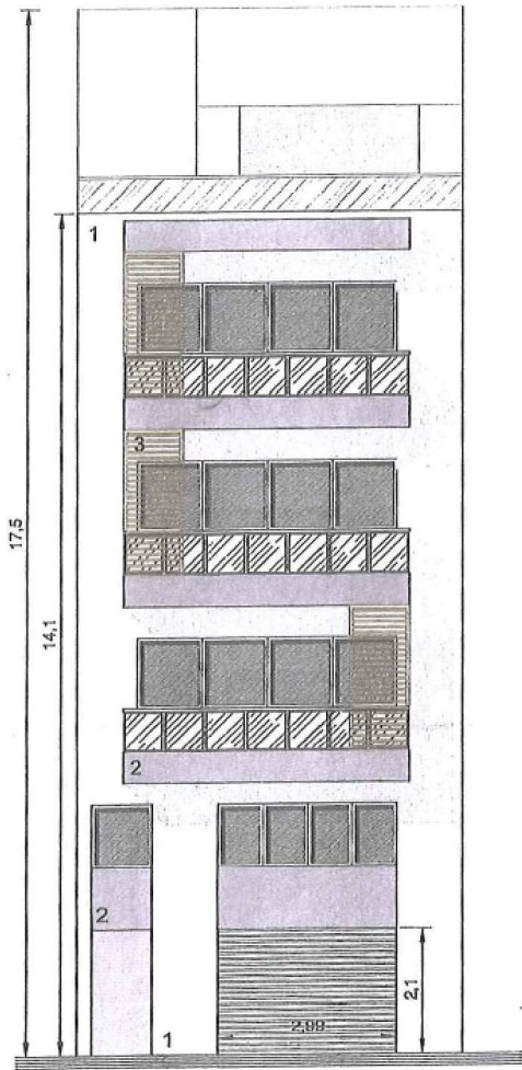
Elevation A
